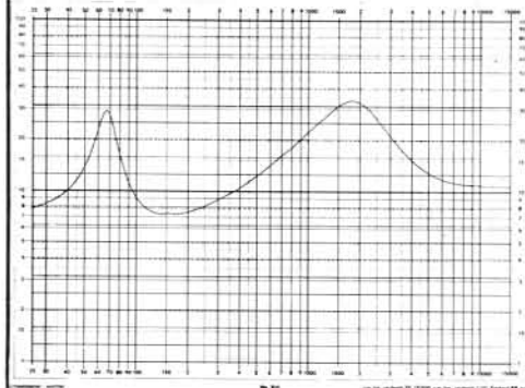
Impedantiekromme van de Impact 1.
